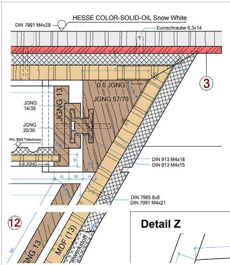
Technische Zeichnung, erstellt mit PYTHA - präzise Planung für maßgeschneiderte Lösungen.
